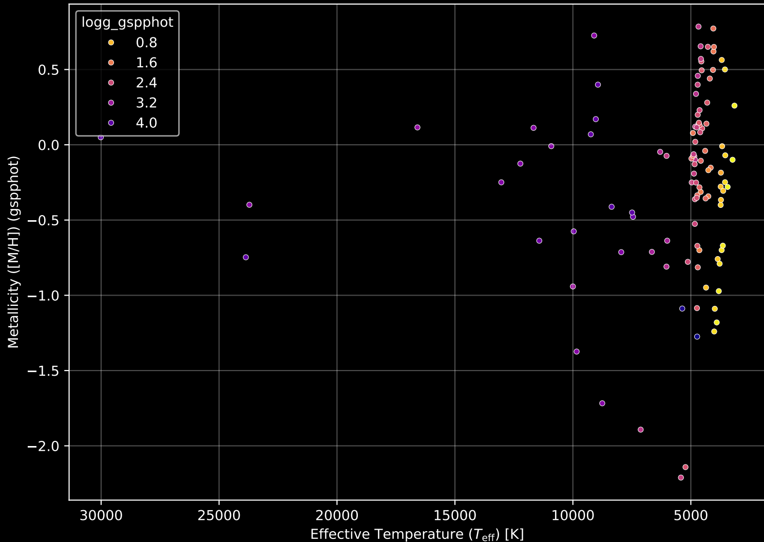
APOGEE DR17 Field: [001-01] Stellar Population Parameters (n= 106)
